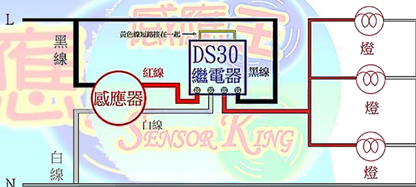
感應器(AC)高負載燈具接線圖
